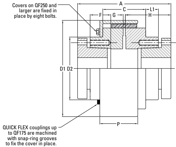
Fig. 24. QUICK FLEX QD style hubs.
