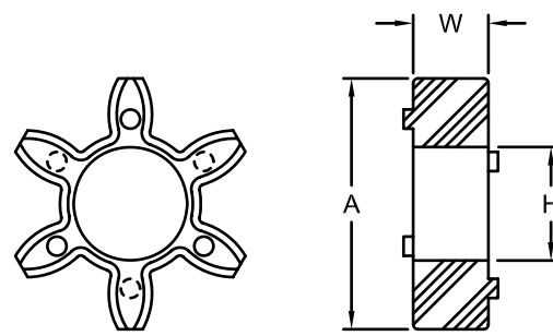
CJ 19/24
