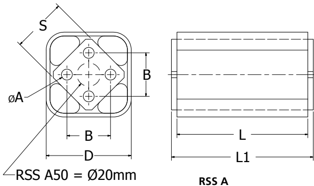
RSS A
