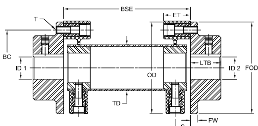
Model 6 (Zytel®)
