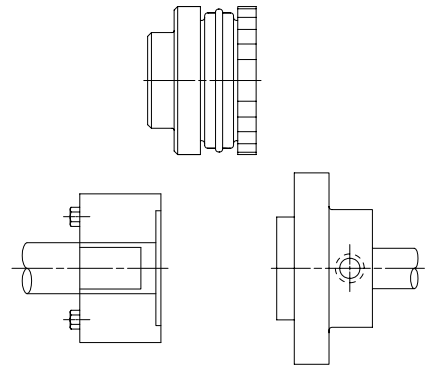
Semi-Spacer
