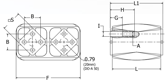
RSD A50
