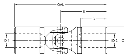
NB Type
