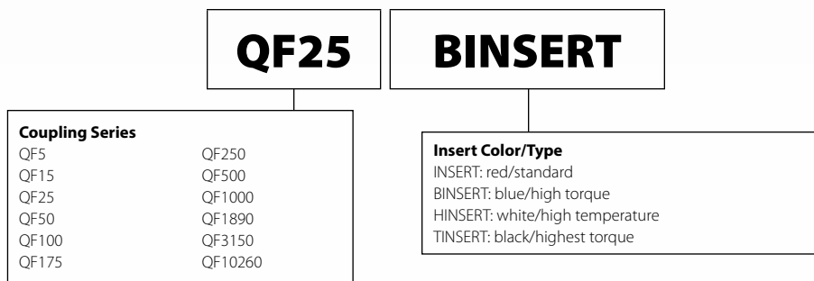
Fig.2. Inserts
