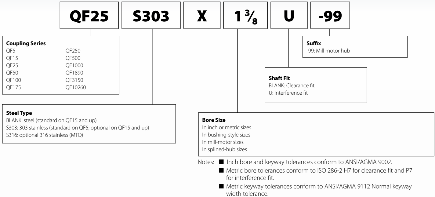
Fig. 1. Hubs
